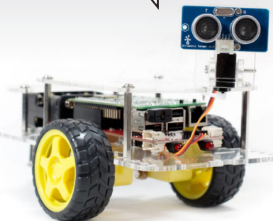
GoPiGo Robot Raspberry Piを利用したロボット組立キット
